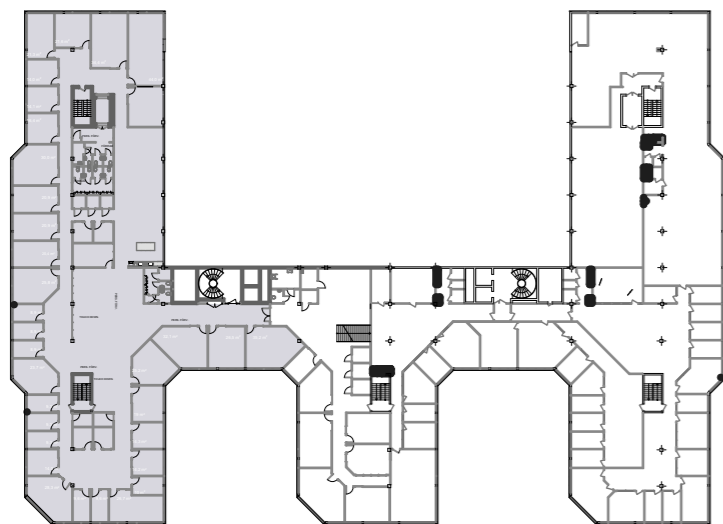
ÖVERSIKTSPLAN 1:1000
