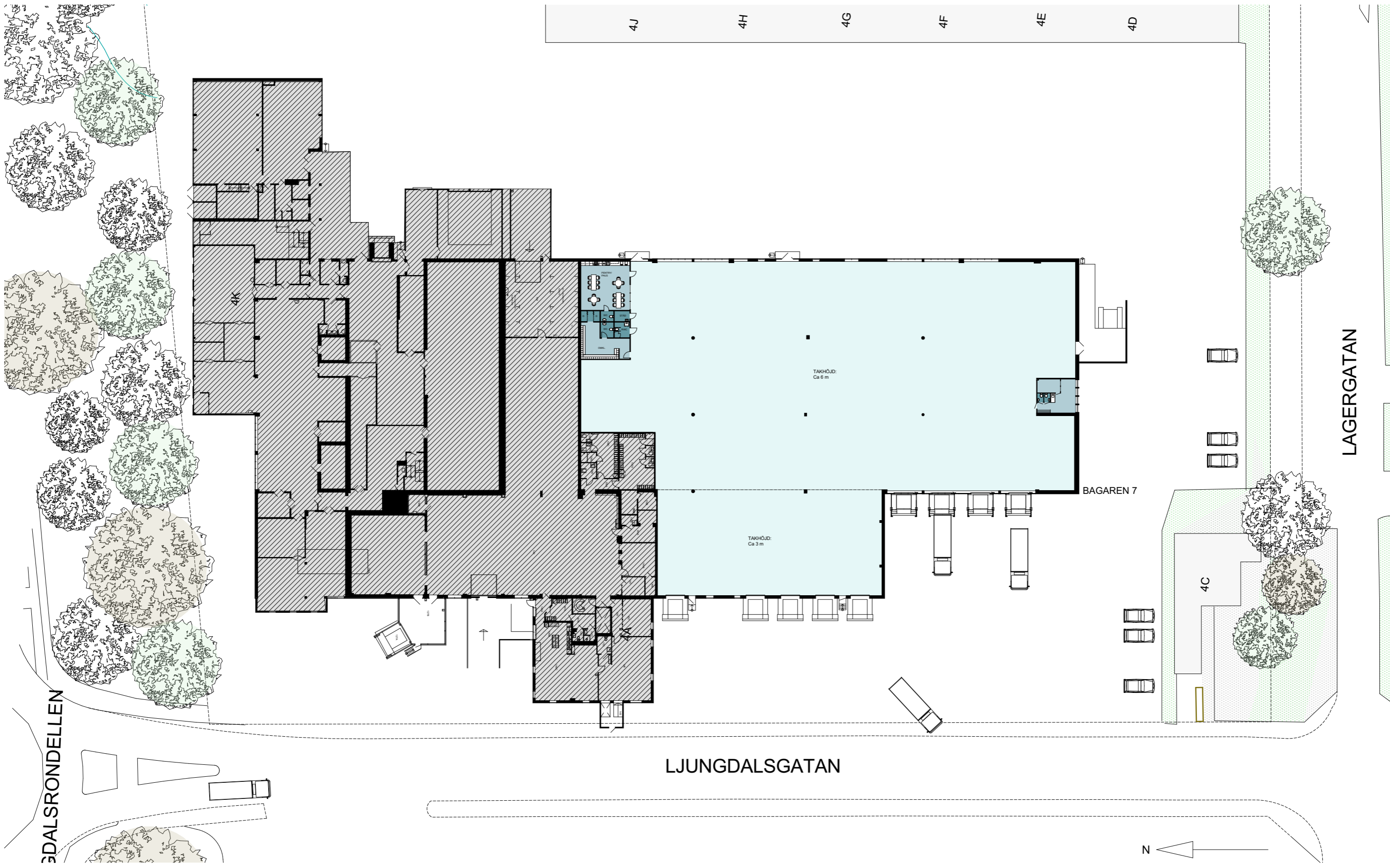
KV. BAGAREN 7 - FÖRSLAG HYRESGÄST DEL AV PLAN 1 - YTA ~ 2725m 2 ILLUSTRATIONSRITNING SKALA A31:500 - 2017-05-11
