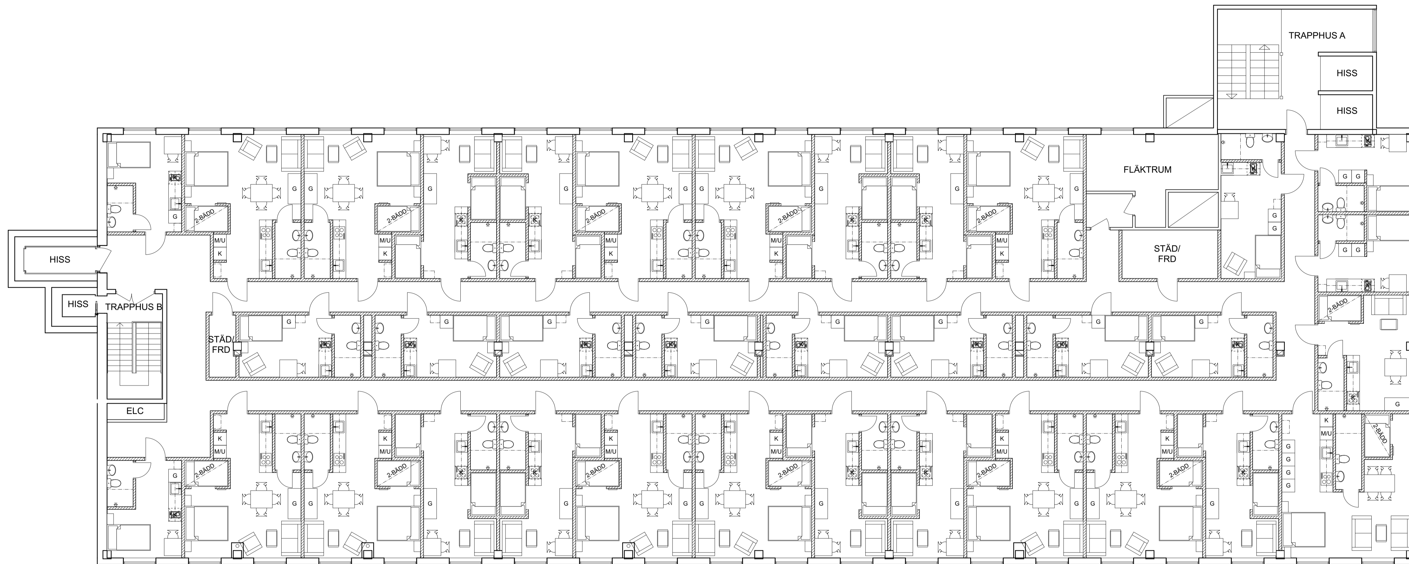
PLAN 4 YTA 1.123 kvm
